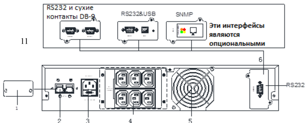
Рис. 2-2 Возможные конфигурации задней панели ИБП HR1101S (L)
