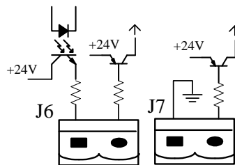
Рисунок 2-14Разъем ВСВ
