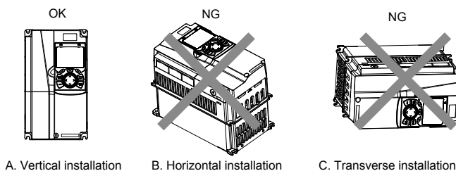
Рис 4.1 Установка ПЧ
